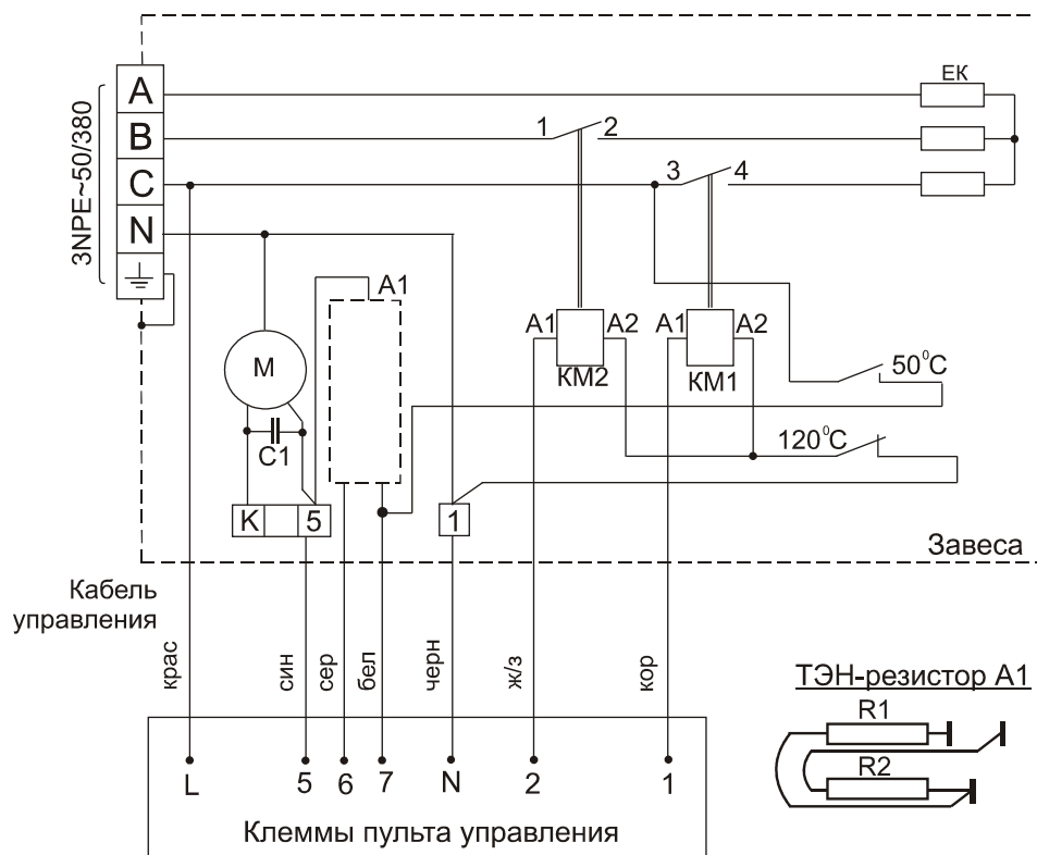
Рис. 3. Электрическая схема КЭВ-9П201Е
