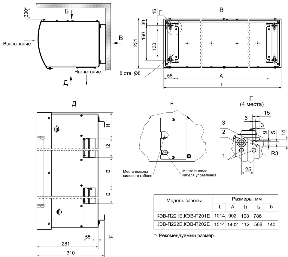
Рис. 7. Крепежные размеры
