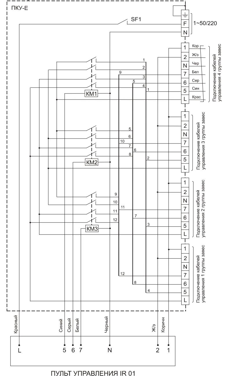
Рис. 6. Электрическая схема ПКУ-Е
