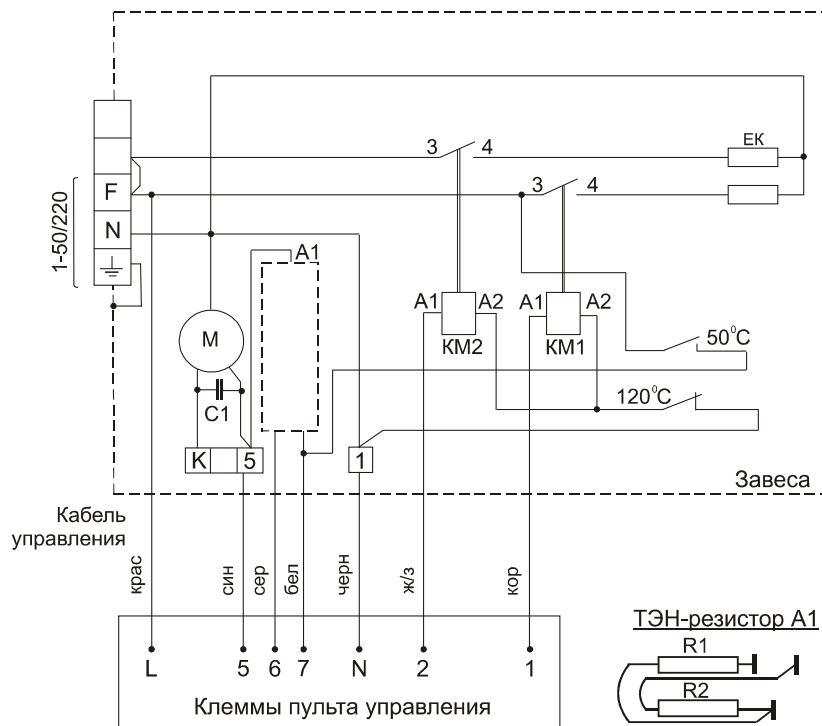
Рис. 1. Электрическая схема КЭВ-6П221Е
