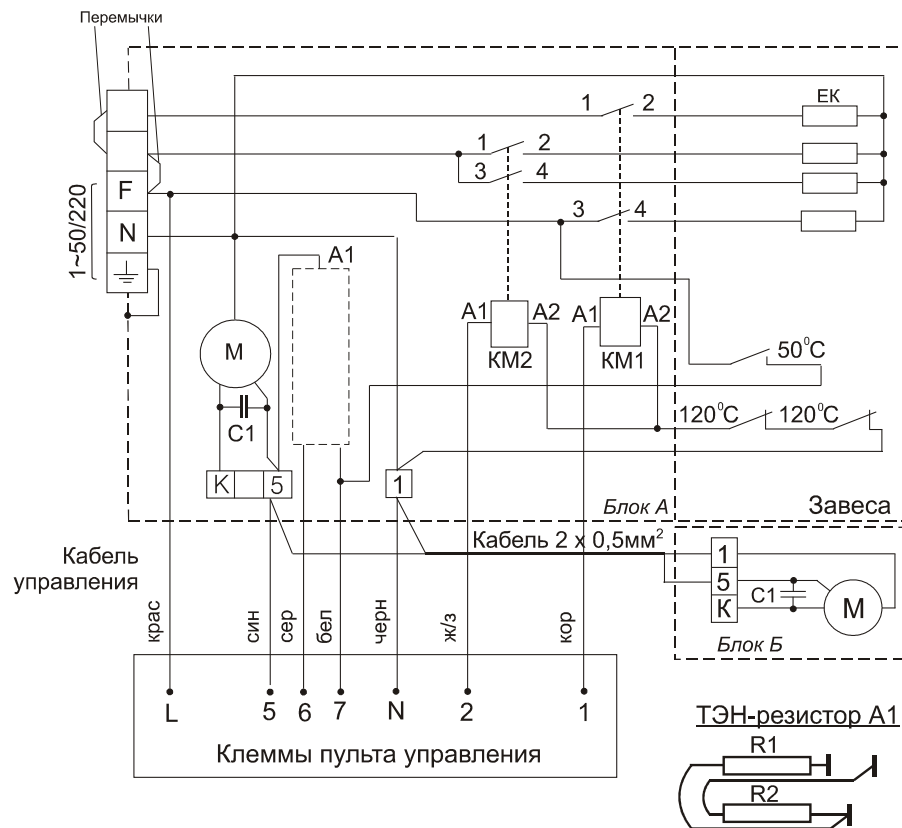
Рис. 2. Электрическая схема КЭВ-6П222Е
