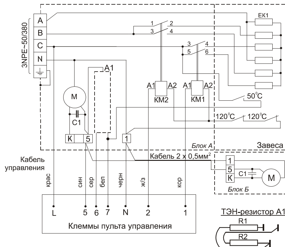
Рис. 4. Электрическая схема КЭВ-9П202Е, КЭВ-12П202Е
