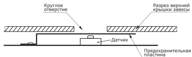
Рис. 9. Аварийный термовыключатель
